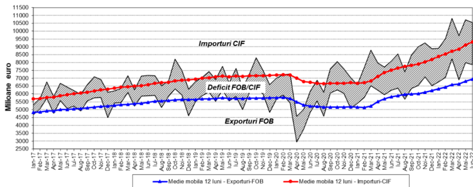
Figura 1: Exporturile, importurile si soldul balantei comerciale FOB/CIF in perioada ianuarie 2017 – iunie 2022
