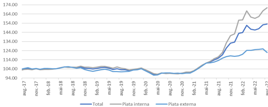
Figura 1: Indicele anual al preturilor productiei industriale pe total, piata interna si piata externa (%)
